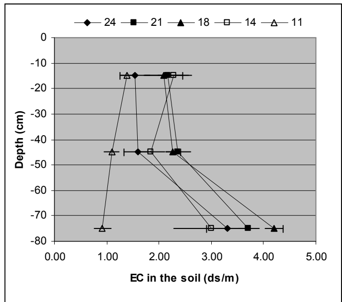
איור 5: המוליכות החשמלית \pm שגיאת תקן בפרופיל הקרקע ב-27 יולי 2008 בחמשת טיפולי ההשקיה. מספרי הטיפולים מציינים את קריאות היעד בתא הלחץ (בר).
